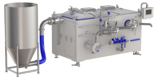
QuadrocultVac 225 - TemBi
