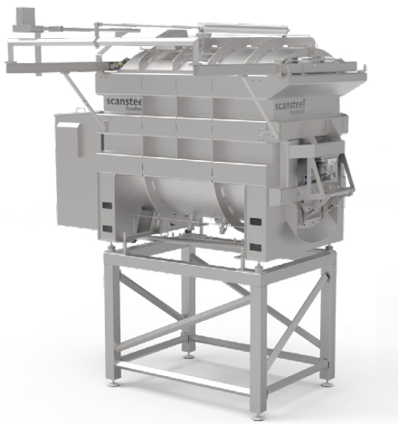
scanDefrost 6000 L.
